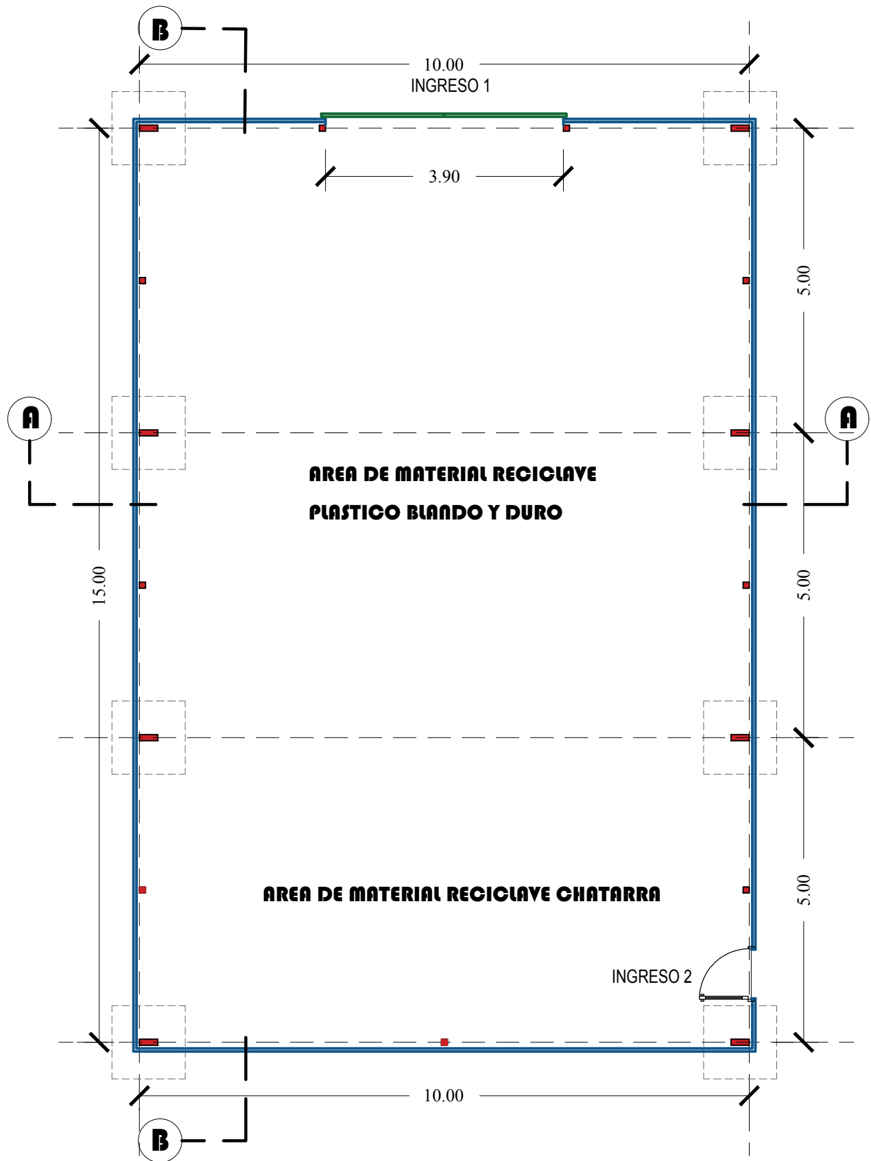
PLANO EN PLANTA ESCALA 1/75
